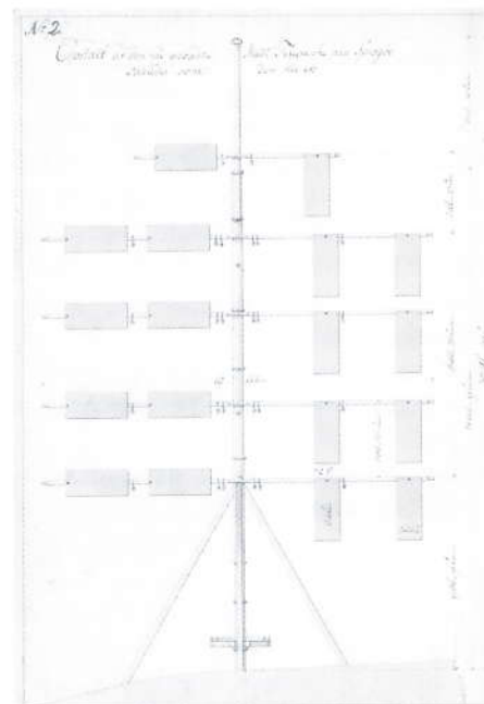
Skitse til en telegraf af Lorentz H. Fisker.
