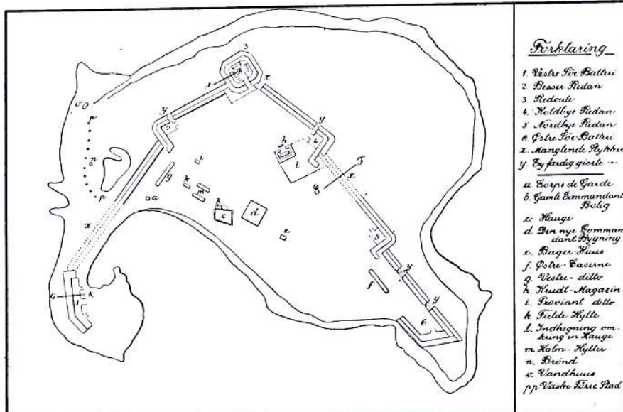
Kort over Kyholm ca. 1807, hvor man ser redouten længst mod nord, de to sobatterier i de sydlige spidser, forbundet med envelopper. Den østlige af disse lige som den vestlige brudt ved to redaner.
